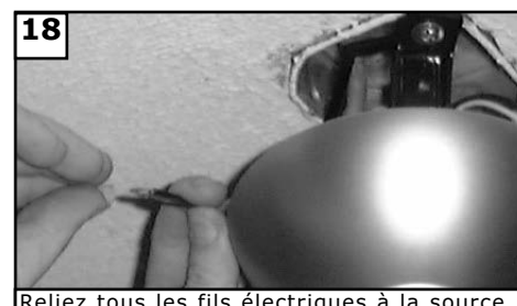
18 Reliez tous les fils électriques à la source d'énergie en utilisant les capuchons électriques fournis à cet effet. Assurez-vous qu'aucun filament ne dépasse des capuchons électriques. Après avoir établi les liaisons électriques, vous devez étaler les fils en mettant le conducteur mis à la masse et le conducteur de mise à la terre de l'appareillage d'un côté du boîtier de sortie de courant et le conducteur non mis à la terre de l'autre côté de la boîte de sortie de courant.
