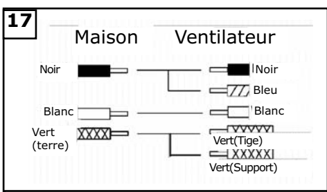
17 Pour la commande du ventilateur par la tirette, suivre le schéma ci-dessus. S'assurer que toutes les parties exposées des fils électriques sont couvertes par les capuchons électriques. Remarque: la couleur des fils électriques de l'installation centrale peut être différente et il est possible que l'installation ne comprenne pas de fil de terre. Une fois le branchement terminé, repousser doucement les fils électriques dans la boîte de raccordement, les capuchons électriques pointés vers le haut. Se reporter au point 3 des conseils de sécurité.
