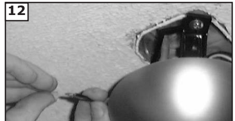
12 Reliez tous les fils électriques à la source d'énergie en utilisant les capuchons électriques fournis à cet effet. Assurez-vous qu'aucun filament ne dépasse des capuchons électriques. Après avoir établi les liaisons électriques, vous devez étaler les fils en mettant le conducteur mis à la masse et le conducteur de mise à la terre de l'appareillage d'un côté du boîtier de sortie de courant et le conducteur non mis à la terre de l'autre côté de la boîte de sortie de courant.
