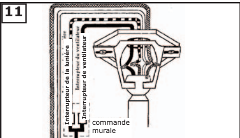
11 Pour la commande murale du ventilateur et du kit d'éclairage optionnel, suivre le disgramme ci-dessus. REMARQUE: Il est recommandé démployer les services d'un électricien qualifié pour ce genre d'installation.
