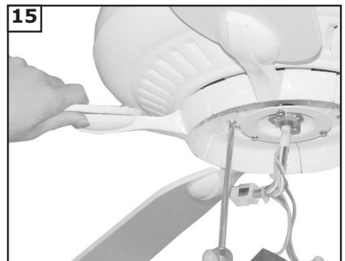
15 Inspecter le moteur pour trouver des pattes stabilisatrices en plastique pour le transport, et les enlever, le cas échéant. Fixer l'ensemble de la pale au moteur avec les vis à moteur et rondelles fournies. Bien serrer les vis.
