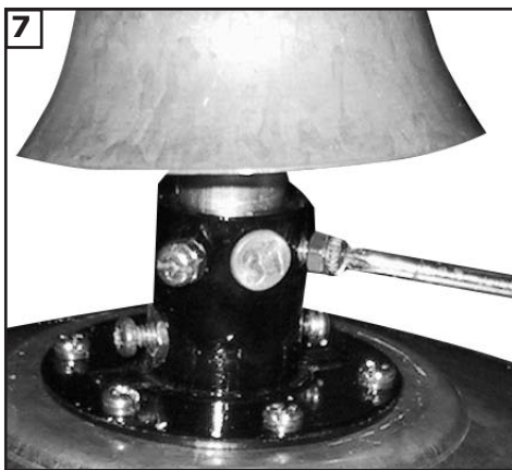
7 Attacher fermement la tige-cache en serrant les deux vis sans tête présentes sur l'embout.
