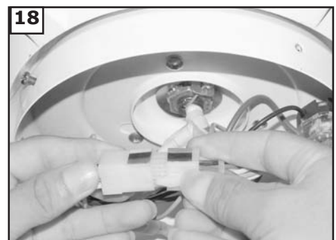
18 Raccorder la fiche du ventilateur à la prise de la plaque de boîtier d'interrupteur.
