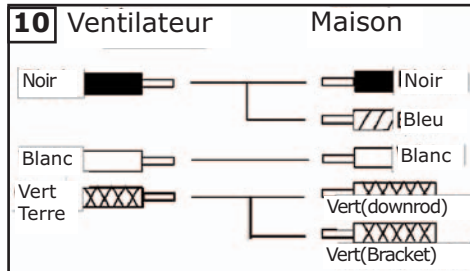
10 Ventilateur Maison Pour la commande du ventilateur par la tirette, suivre le schéma ci-dessus. S'assurer que toutes les parties exposés des fils électriques sont couvertes par les capuchons électriques. Remarque: la couleur des fils électriques de l'installation centrale peut être différente et il est possible que l'installation ne comprenne pas de fil de terre. Une fois le branchement terminé, repousser doucement les fils électriques dans la boîte de raccordement, les capuchons électriques pointés vers le haut. Se reporter au point 3 des conseils de sécurité.
