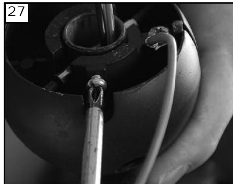
27 Serrer la vis de réglage pour tenir la sphère en place.
