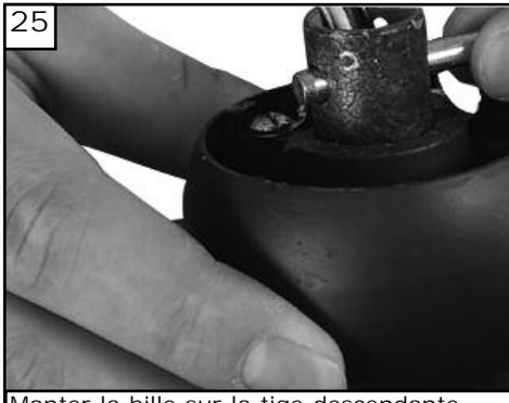
25 Monter la bille sur la tige descendante. Remettre en place la goupille enlevée précédemment de manière à ce qu'elle pénètre dans les fentes de la bille.
