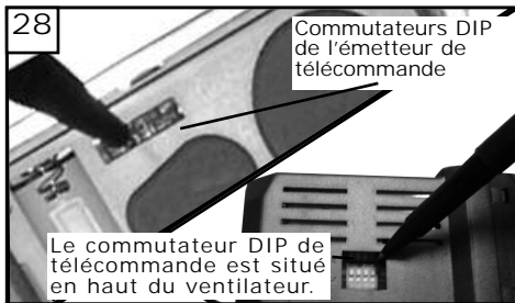
28 Réglez les commutateurs DIP sur l'émetteur de télécommande et sur le récepteur de télécommande sur les mêmes commandes. Ceci est obligatoire si vous voulez que les deux unités communiquent correctement. D'autres ventilateurs peuvent être réglés sur un émetteur en réglant les deux récepteurs sur les mêmes commandes que l'émetteur. Si vous avez plusieurs ventilateurs comportant leur propre émetteur, vous pouvez régler les commutateurs DIP sur différentes positions pour pouvoir les commander séparément.
