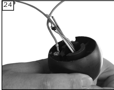
24 Enfiler les fils et le câble de sûreté par la sphère.
